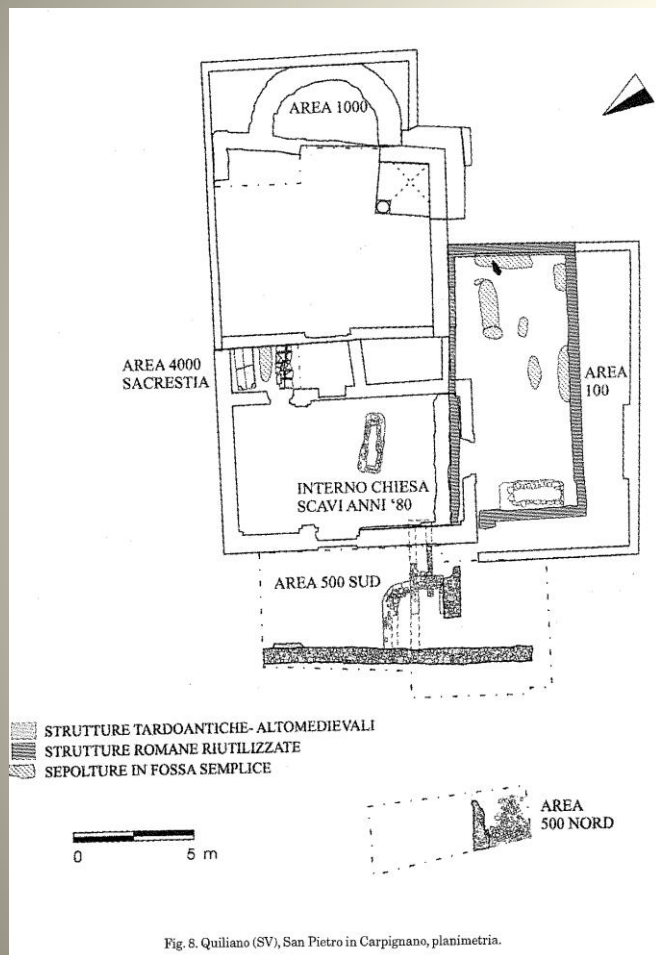
Fig. 8. Quiliano (SV), San Pietro in Carpignano, planimetria.
